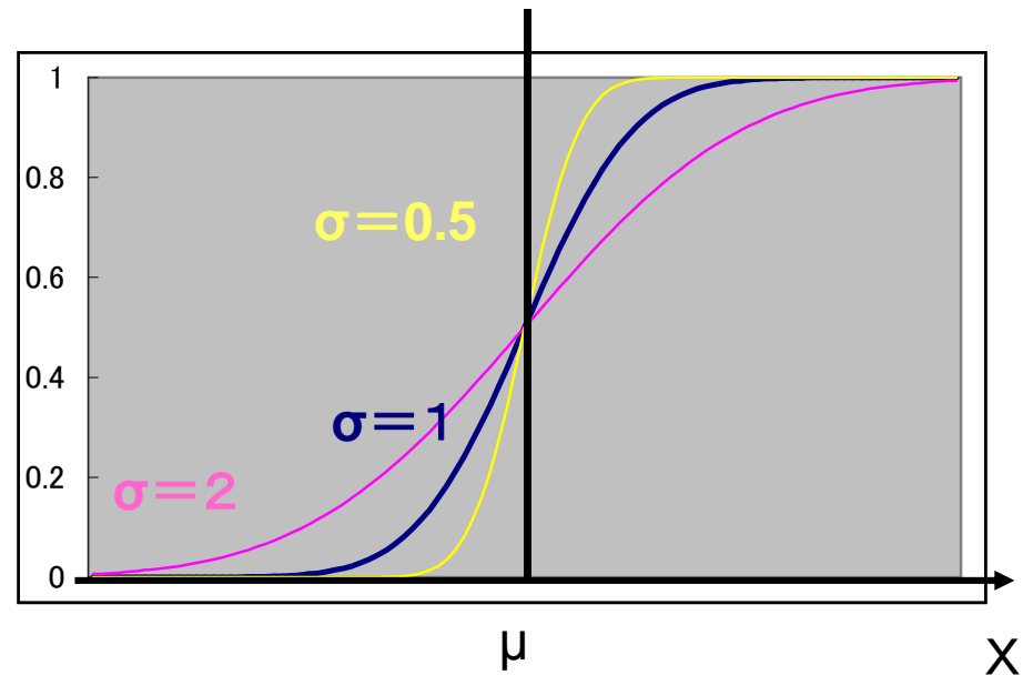
F(X) 分布関数 (累積確率密度関数)
